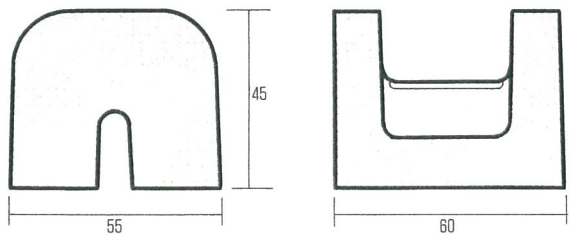
断面形状
